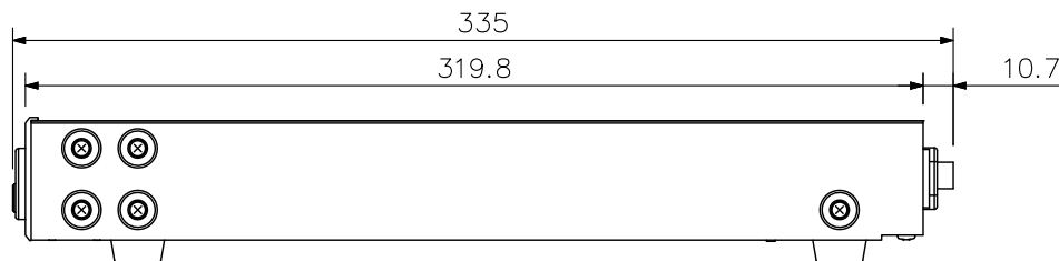
側面図
