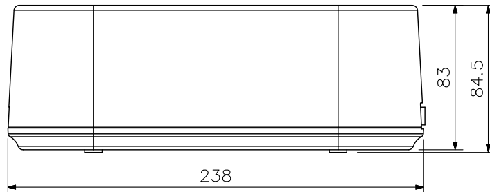
正面図
