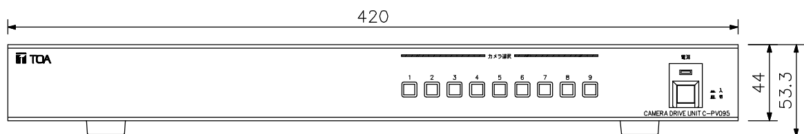
正面図
