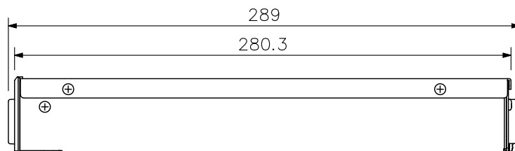
側面図
