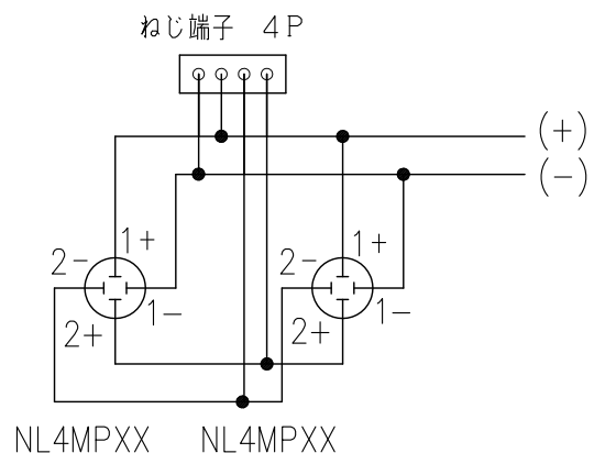
結線図
