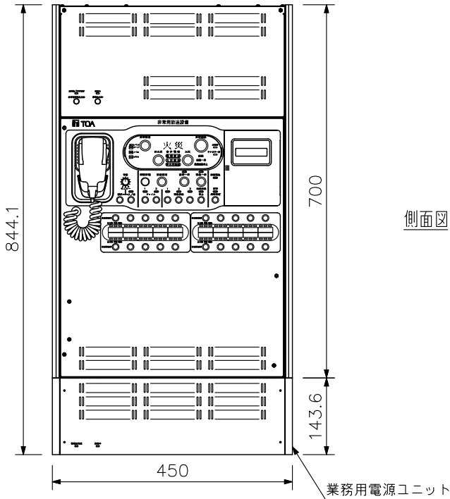
正面図
