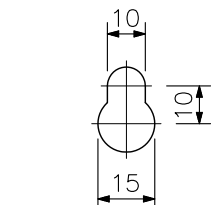
取付穴 (上部左右2カ所) (縮尺: 1/2)
