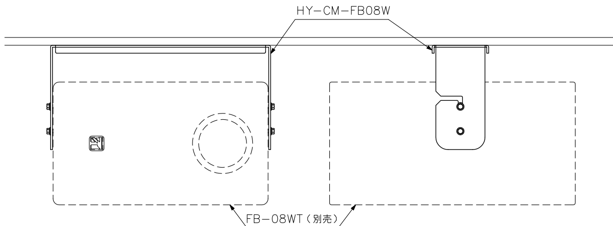
取付例 (縮尺: 1/6)
