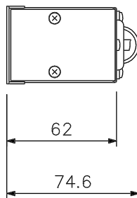
側面図
