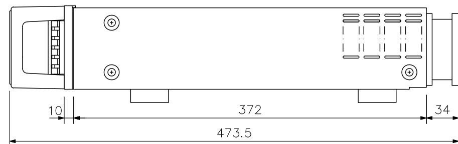
側面図
