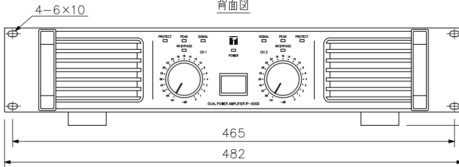
正面図
