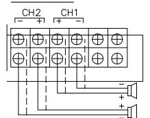
出力端子部
