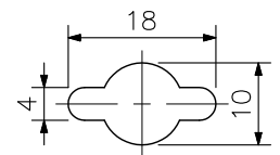
壁取付穴拡大図 (縮尺: 1/1)
