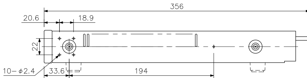
側面図
