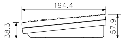
据置図(縮尺: 1/5)
