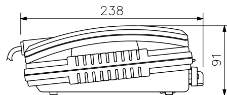
据置図(縮尺: 1/5)
