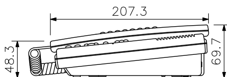
据置図（縮尺：1/5）
