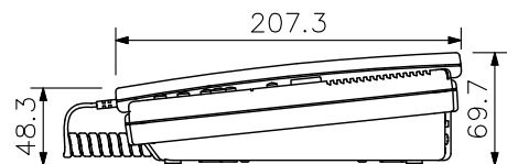
据置図（縮尺：1/5）
