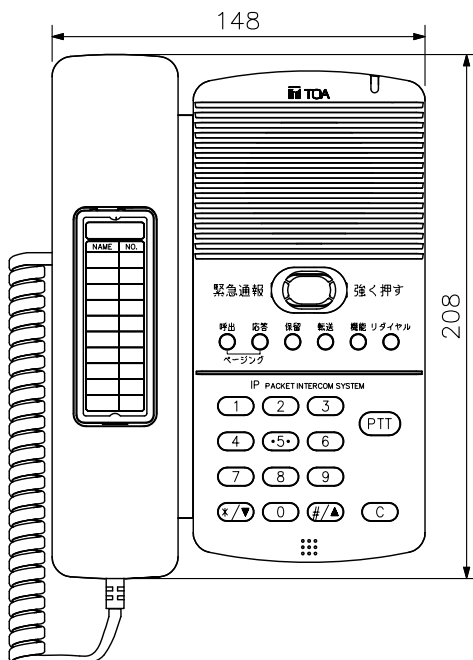
正面図
