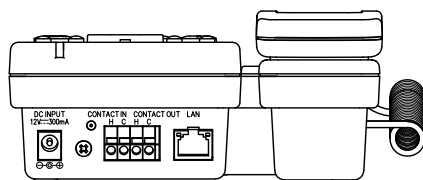
上面図
