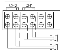
出力端子部
