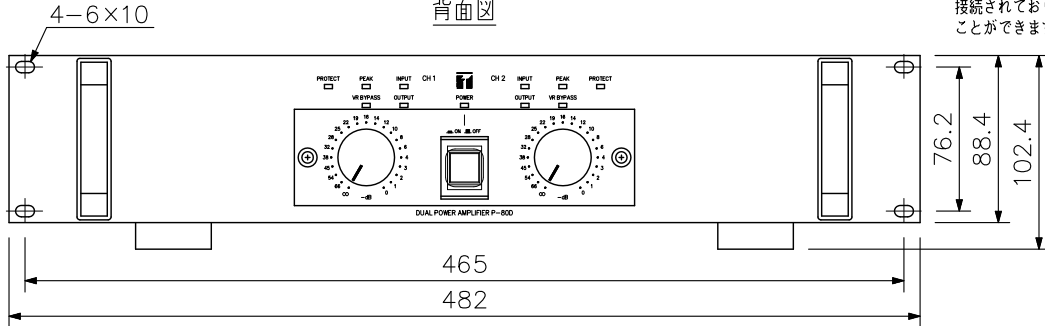
正面図
