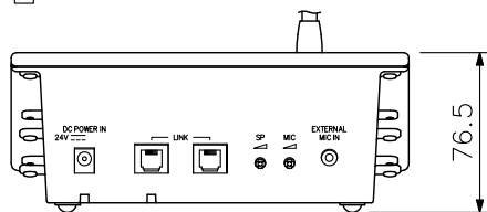
背面図
