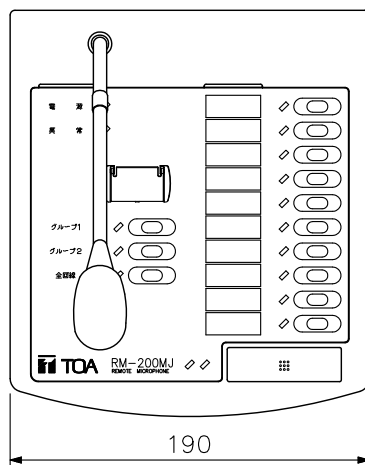
A矢视图
