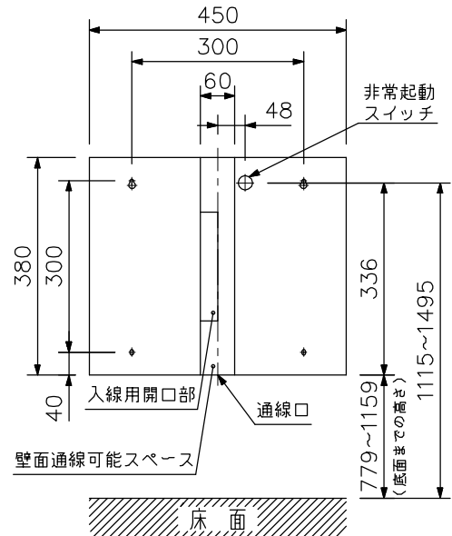
壁取付工事図
