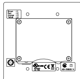
背面図
