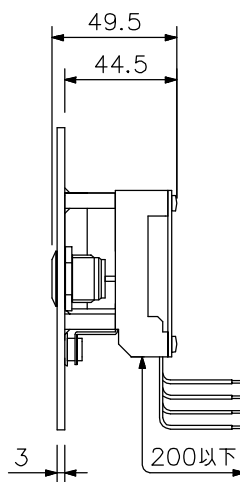
側面図
