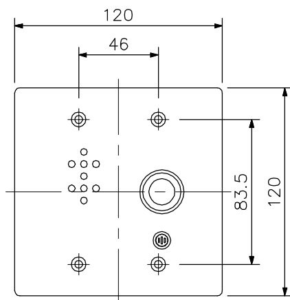
正面図
