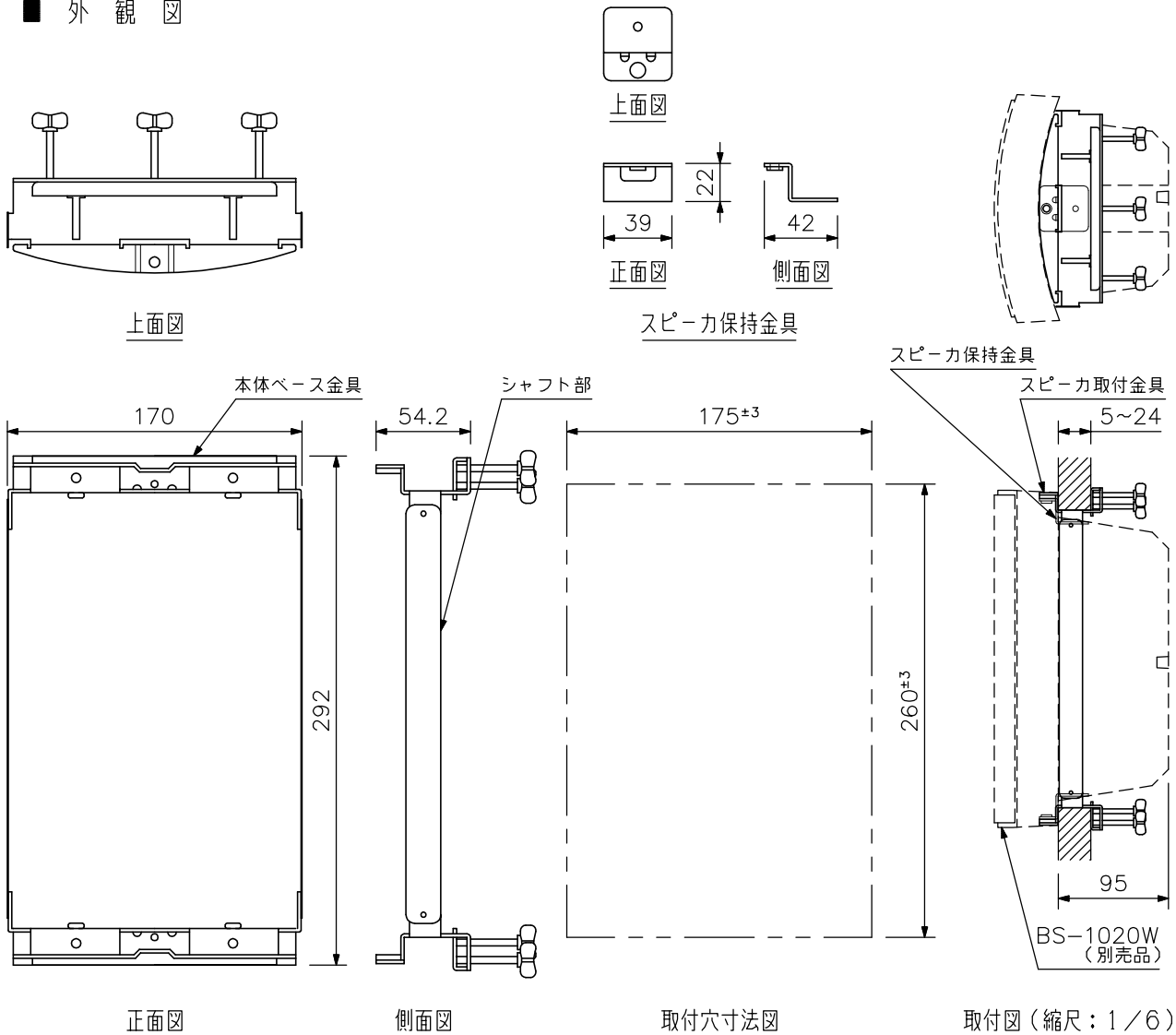
スピーカー取付金具(蝶ボルト付)
