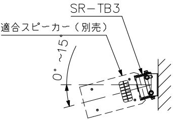
取付例 (上面図) (縮尺: 1/10)
