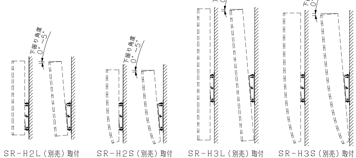
取付例 (縮尺: 1/20)
