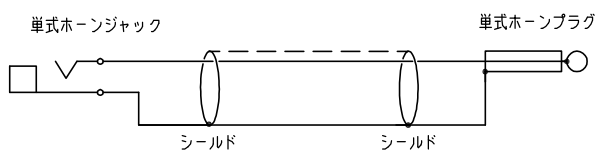
回路図
